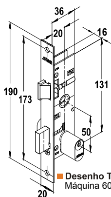
Desenho Técnico Máquina 501/502/503
