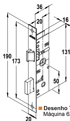
Desenho Técnico Máquina 601/602/603
