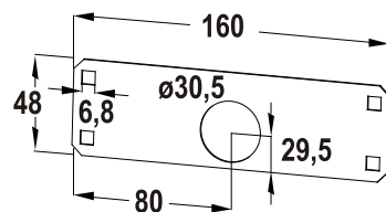
■ Desenho Técnico Espelho 201/1201
