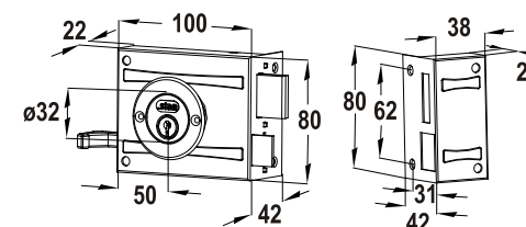
Desenho Técnico Máquina 701/100
