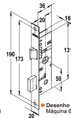
Desenho Técnico Máquina 601/602/603
