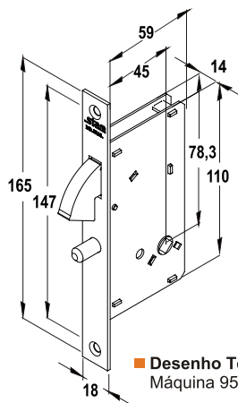
Desenho Técnico Máquina 950/955
